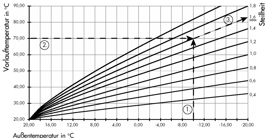
Heizkennlinien
