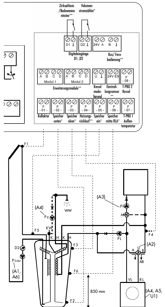
Anschluss-Schema
