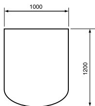
Korbbogen- Funkenschutzplatte
