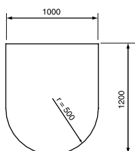
Rundbogen- Funkenschutzplatte
