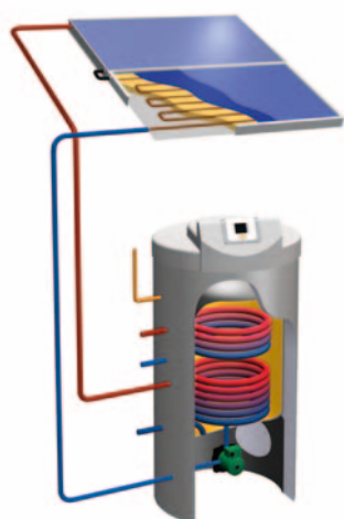
SECUSOL 250-2 Solarkompaktsystem zur Warmwasserbereitung
